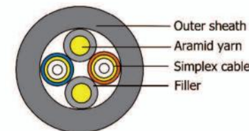
FTTA Cable
