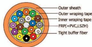
Breakout Cable
