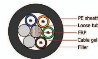
GYFTY Cable
