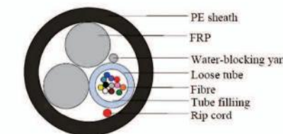
ASU Cable
