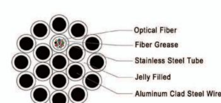
OPGW Cable
